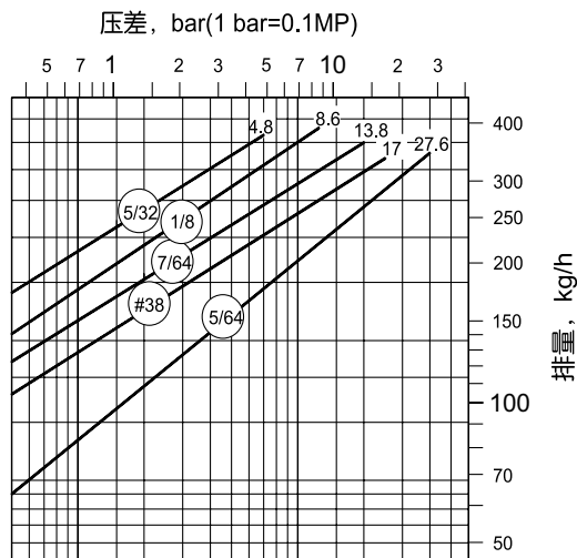
2011 型疏水阀排量图
