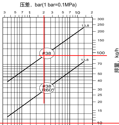
2010 型疏水阀排量图
