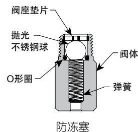
防冻塞
