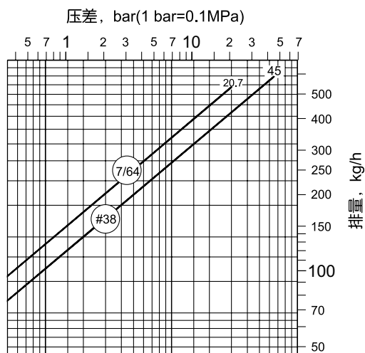
2022 型疏水阀排量图
