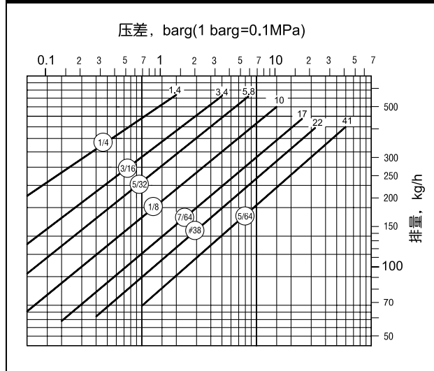
981 型排量图
