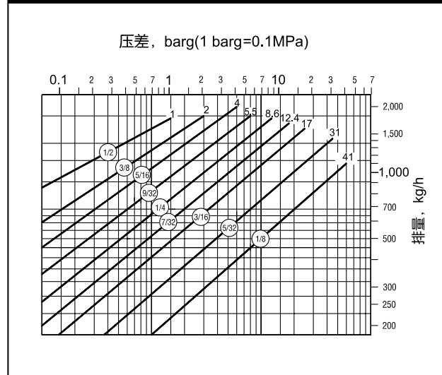
983 型排量图
