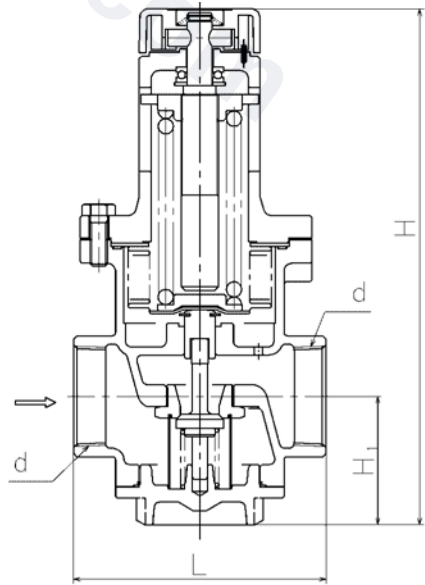
DN40、DN50
