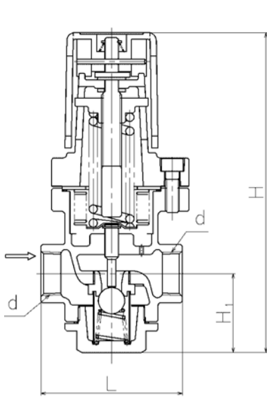
DN15、DN20、DN25
