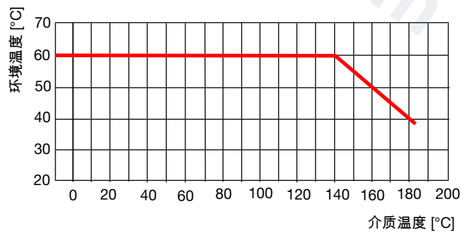
图 6: 温度范围，PA 执行机构，执行机构尺寸 50 (D)
