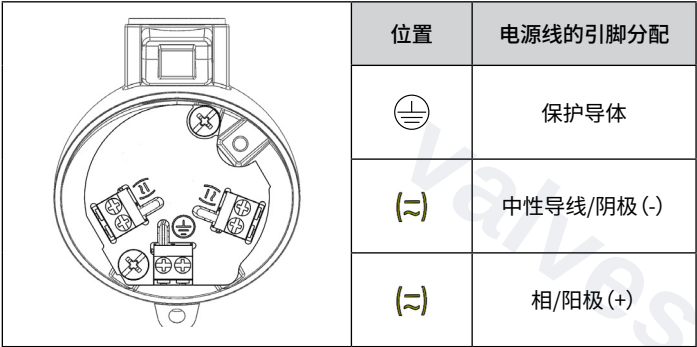
图8： 接线盒
