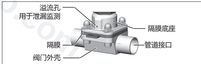
图片 29：溢流孔
