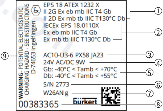
图4: 防爆铭牌的位置和说明 (示例)
