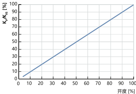
线性流量特性曲线——各个阀座公称尺寸的 K_{vs} 值均可在章节“6.2. 压力范围”在第 10 页中找到。
