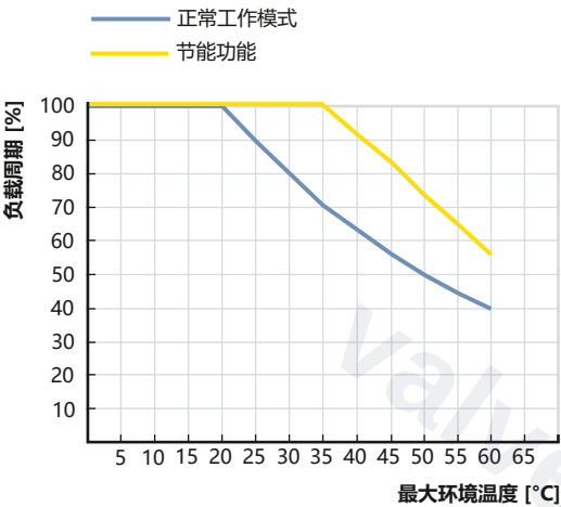
针对标准设备的降额曲线
