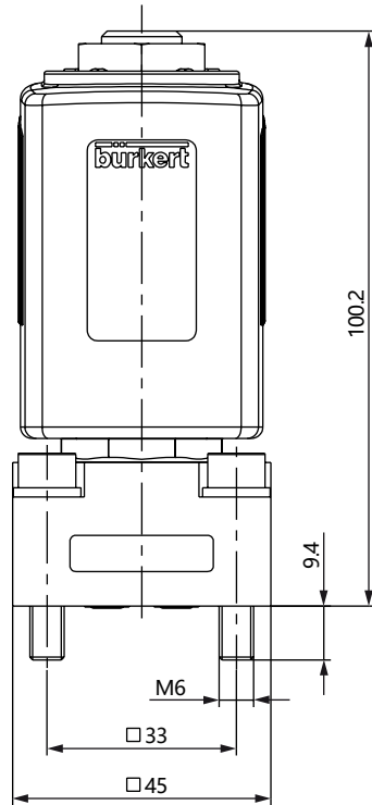
连接尺寸图
