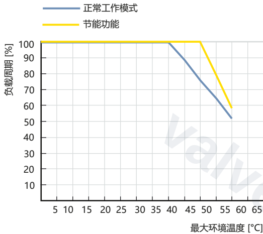
3280 型 阀座 DN1~6 < 6 bar 标准型
