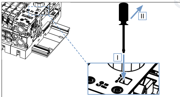
图25: 解锁内藏的解锁滑块
