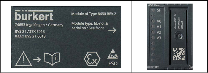
图13： 常规标签 (左侧面)
