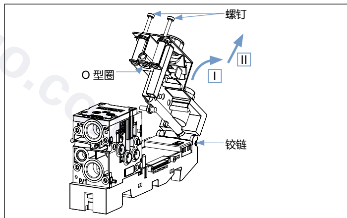
图27: 拆下/安装压力计
