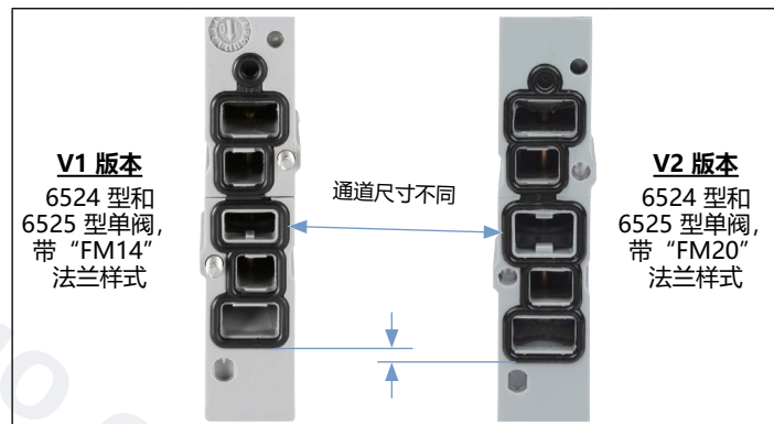
图17: 6524 型和 6525 型单阀的法兰样式差异
