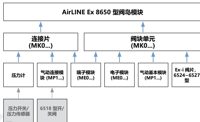
图6： AirLINE Ex 阀岛模块的结构装配来自模块和“基座”
