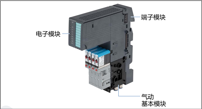
图9: AirLINE Ex V2 版本阀岛模块的阀块单元
