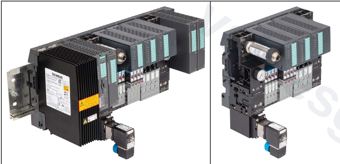
图1： 阀岛视图（Siemens SIMATIC ET 200iSP 和 Bürkert AirLINE Ex）
