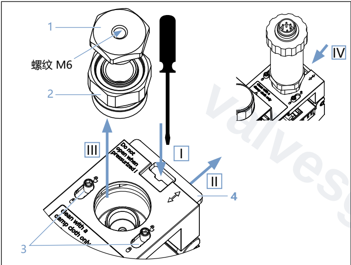
图31: 安装/拆卸连接片上的压力开关/压力传感器
