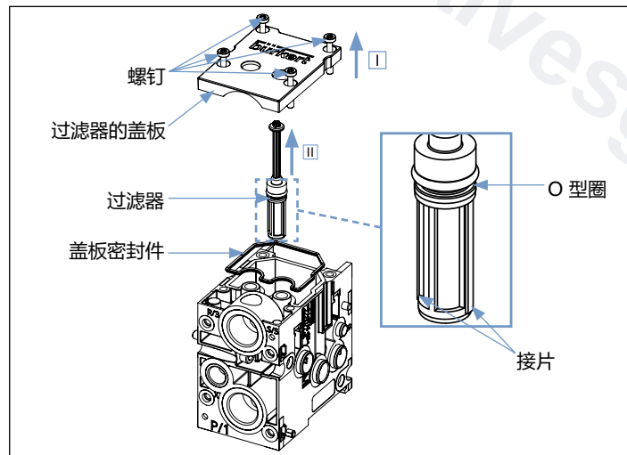
图28: 拆下/安装过滤器
