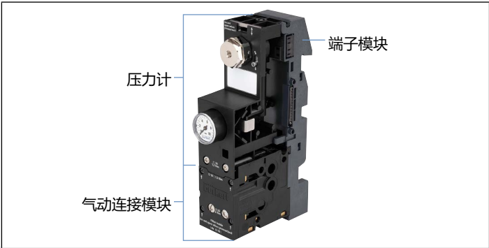
图8: AirLINE Ex V2 版本阀岛模块的连接片
