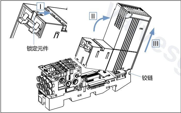
图29： 拆卸/安装阀块单元
