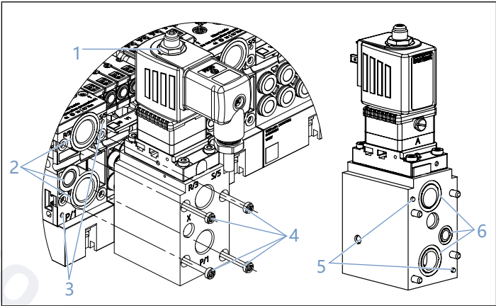
图30： 安装/拆卸开/关阀
