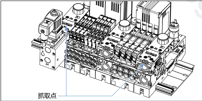
图19： 取出已组装系统的抓取点
