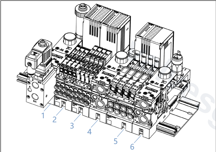
图7: 整个 AirLINE Ex, V2 版本阀岛模块的结构 (示例)
