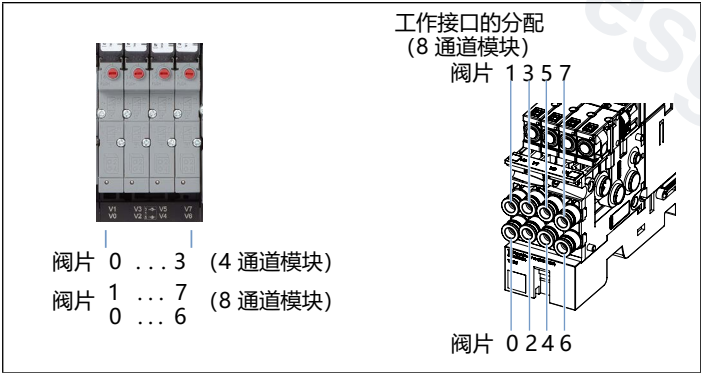
图12： 将工作接口分配到阀片
