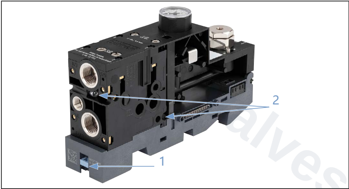
图22： 基座和解锁滑块的斜拉杆
