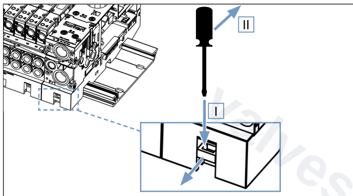
图24: 操作解锁滑块
