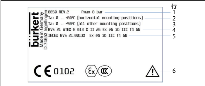
图4： 常规数据铭牌示例
