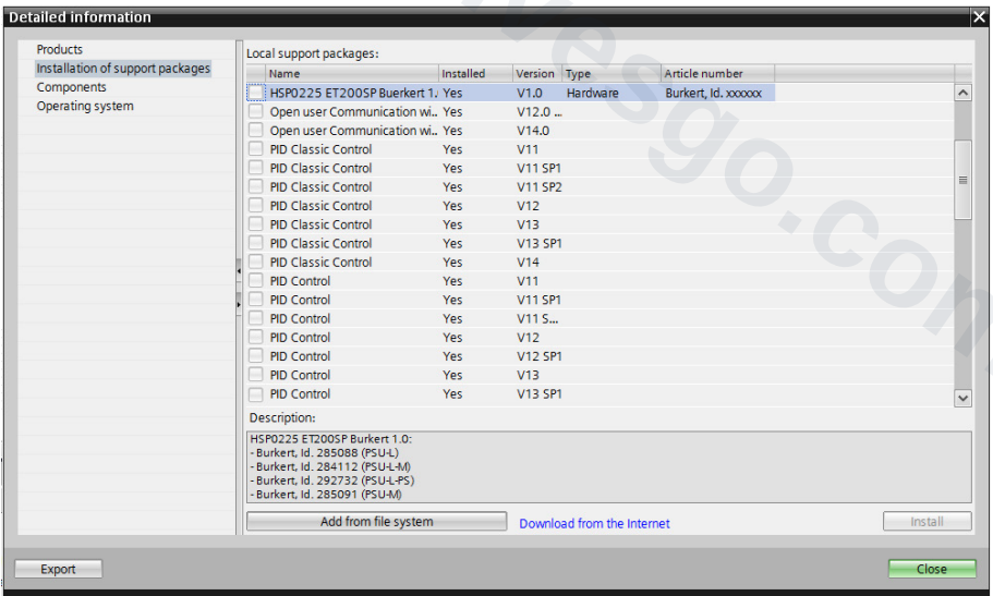
图32: 安装 HSP
