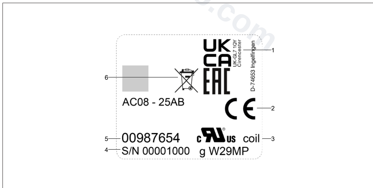
Fig. 3: Type 6211EV laser marking
