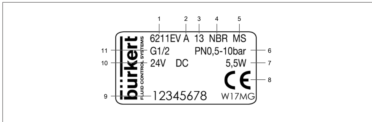
Fig. 2: Type 6211EV type label
