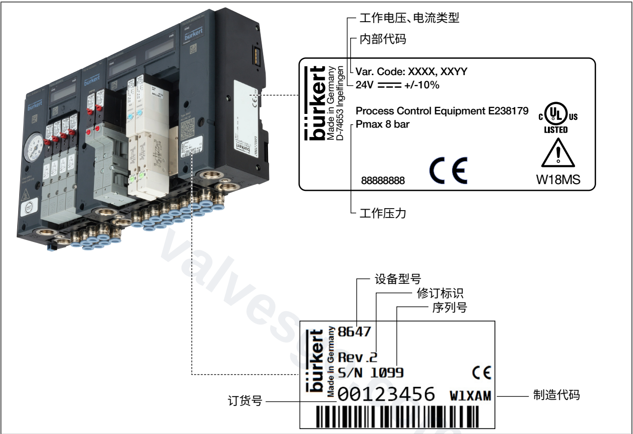
图41: 铭牌的位置和说明 (示例)
