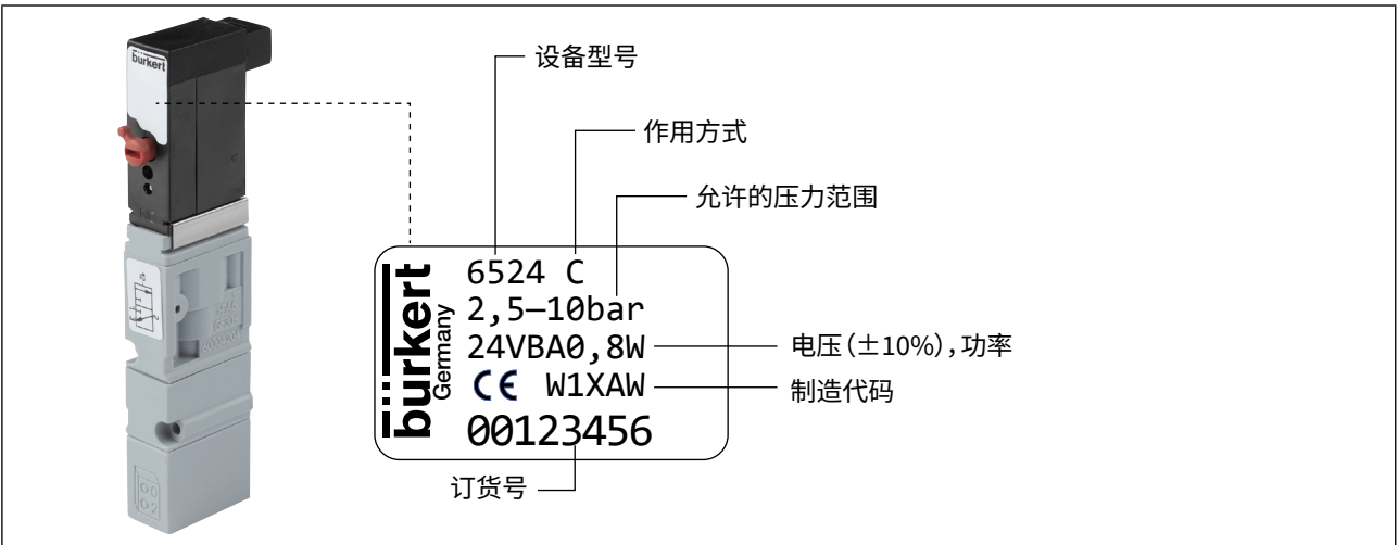
图42: 铭牌的位置和说明 (6524 型示例)
