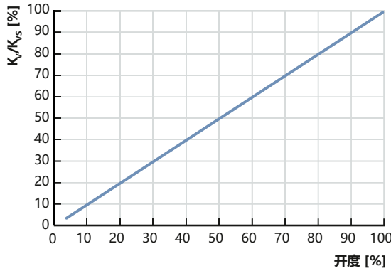
线性流量特性曲线——各个阀座公称尺寸的 K_{vs} 值均可在章节“6.2. 压力范围”在第 13 页中找到。
