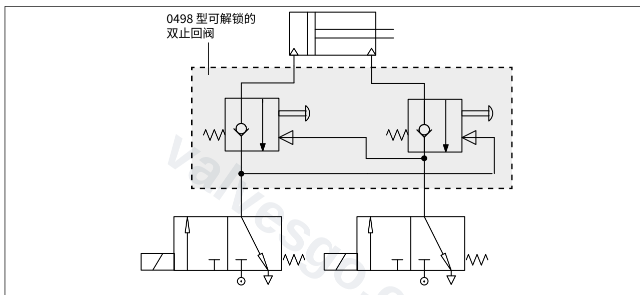
图11: 通过 0498 型阀门和阀块的 2 \times 二位三通阀来运行三位五通功能
