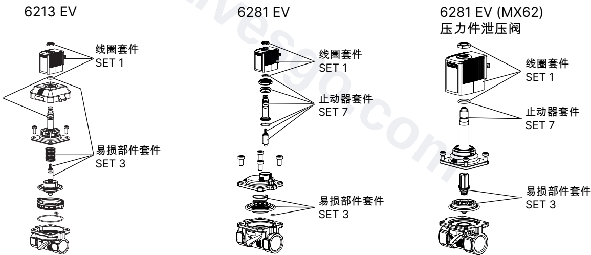
图 1: 备件概述
