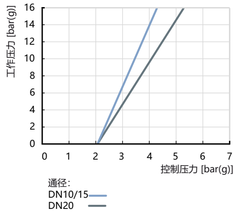
执行机构尺寸 Ø 63 mm (E) 最大控制压力 10 bar(g)
