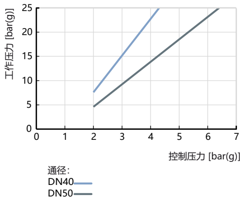
执行机构尺寸 Ø 100 mm (G) 最大控制压力 7 bar(g)
