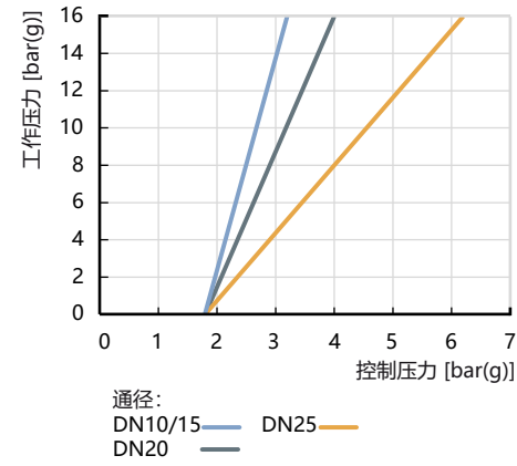
执行机构尺寸 Ø 80 mm (F) 最大控制压力 10 bar(g)
