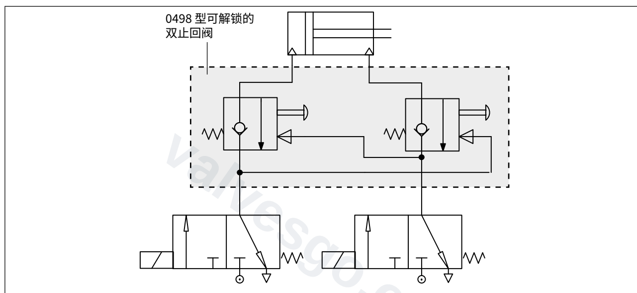
图11: 通过 0498 型阀门和阀块的 2×二位三通阀来运行三位五通功能
