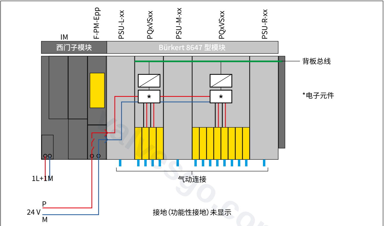
图13: 使用西门子 F-PM-E 模块启动系统
