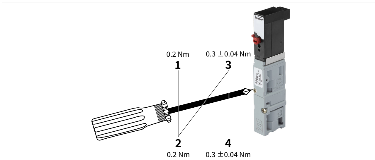
图40: 更换阀门时拧紧螺钉
