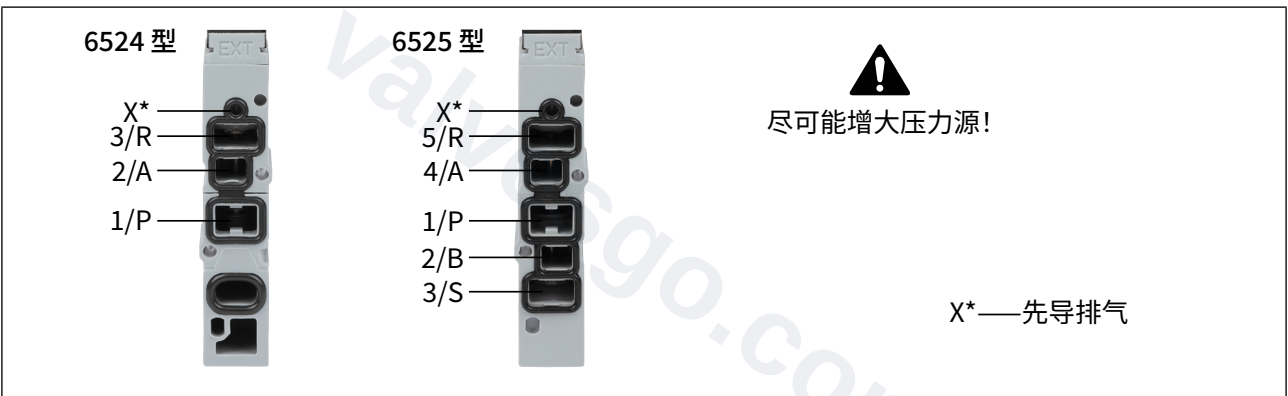
图7： 6524 型和 6525 型单阀流体接口
