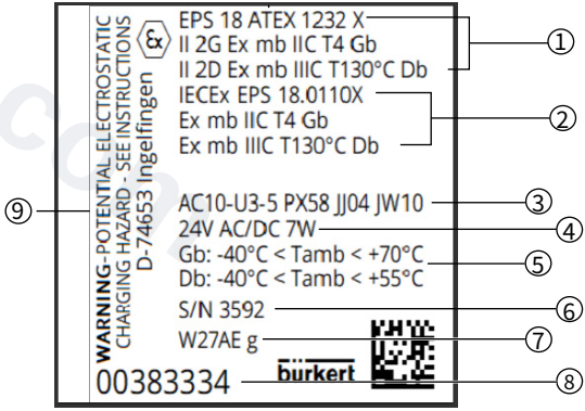
图3: 防爆铭牌的位置和说明(示例)
