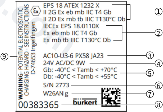
图4： 防爆铭牌的位置和说明 (示例)
