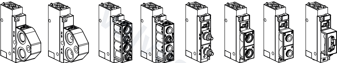
NAMUR 适用于节流螺钉的 版本 B 版本 B 版本 D 版本 E 版本 F 版本 C NAMUR 适用于节流螺钉的 G 1/8 或 气管快插接口 (代码 AF07) NAMUR NPT 1/8 Ø 6 mm
