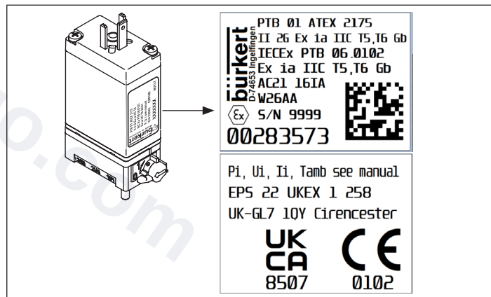
图 1： 铭牌的位置和示例性图示
