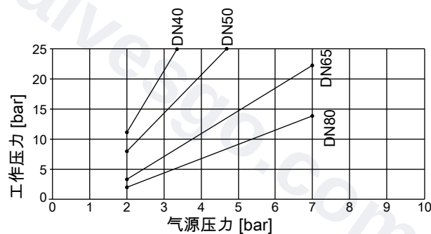
图 17: 最小气源压力, 执行机构尺寸 125 (H), 控制功能 B 和 I
