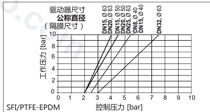
图片 19：控制功能 I、PTFE-EPDM 隔膜、驱动器 Ø 40–63 mm
