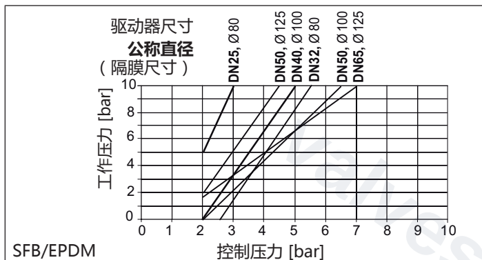
图片 14：控制功能 B、EPDM 隔膜、 驱动器 \varnothing 80–125 mm
