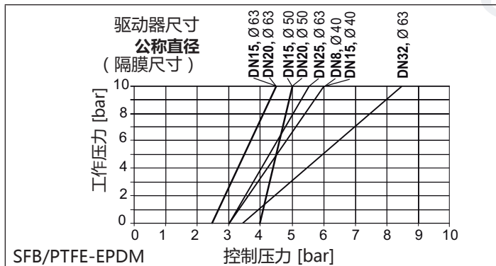
图片 15：控制功能 B、PTFE-EPDM 隔膜、 驱动器 \varnothing 40–63 mm
