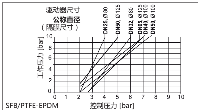
图片 16：控制功能 B、PTFE-EPDM 隔膜、 驱动器 \varnothing 80–125 mm
