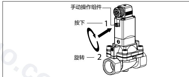
图 2： 手动操作组件
