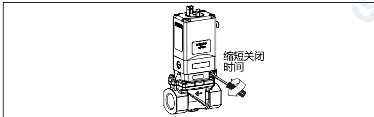
图 6: 缩短 DN13 VA 的关闭时间
