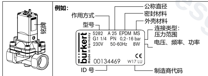
图 1： 铭牌的位置和说明
