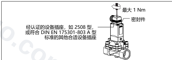
图 7: 设备插座的电气工作接口
