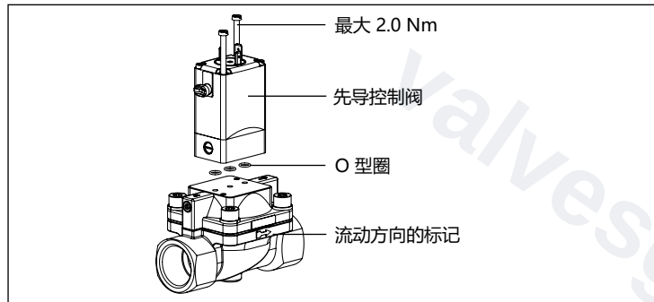
图 3: 安装先导控制阀 (改变阀门功能)
