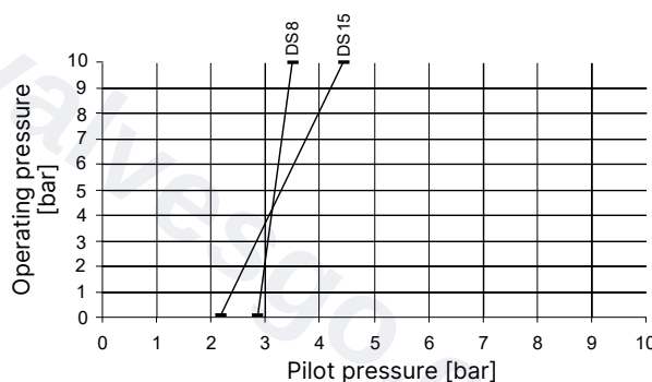
Fig. 10: Control function B, diaphragm material EPDM, FKM, actuator size 50 (D)
