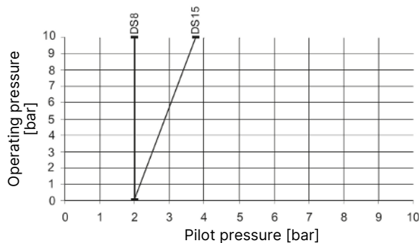
Fig. 26: Control function I, diaphragm material EPDM, FKM, actuator size 50 (D)
