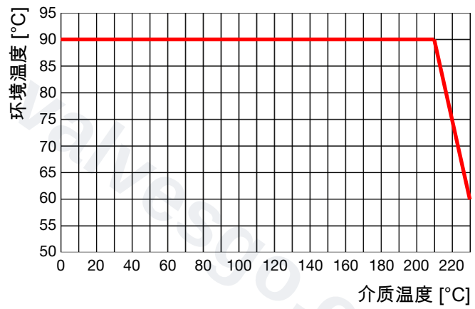
图 10: 衰减，PPS 执行机构，执行机构尺寸 100 (G)、125 (H)
