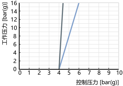
在阀座上流向时的控制压力图(控制功能 A, 阀座密封件 PTFE) 执行机构尺寸 Ø 40 mm 最大控制压力 10 bar(g)
