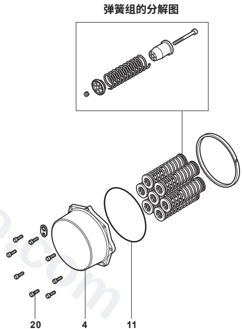
图5. BVA300分解图
