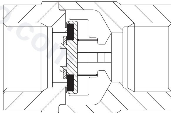
软密封阀座（仅螺纹连接）
