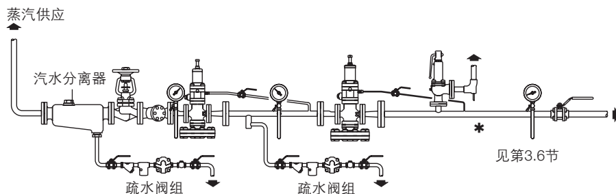
图6 两台减压阀串联安装
