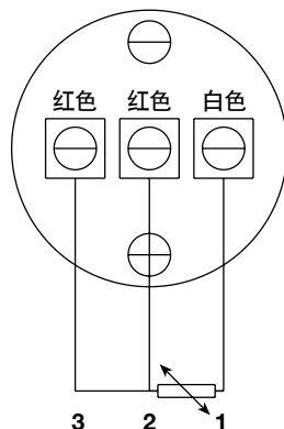
图7 EL2270 接线详图
