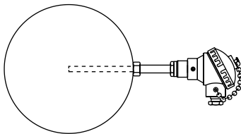
图5 蒸汽系统中推荐安装方式
