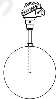
图 6 可接受的安装
