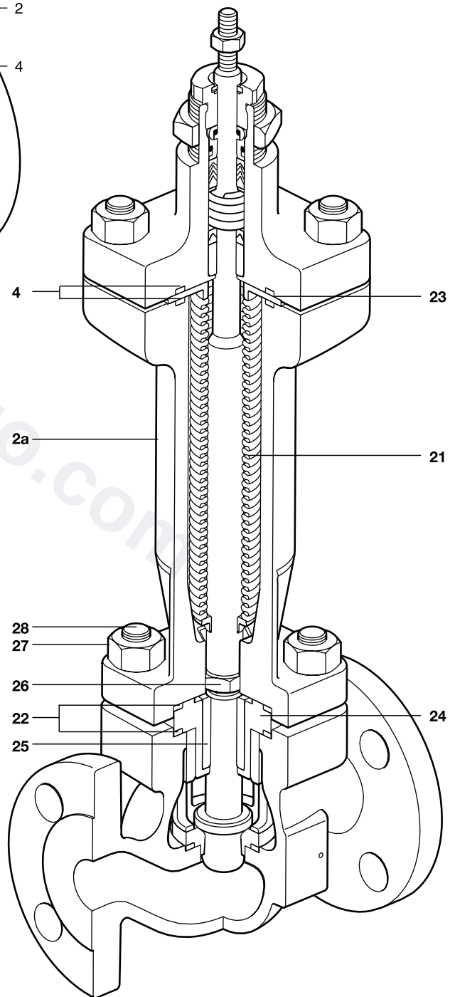
波纹管密封KE73
