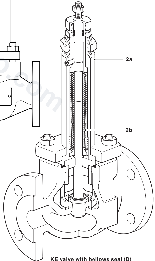
KE valve with bellows seal (D)
