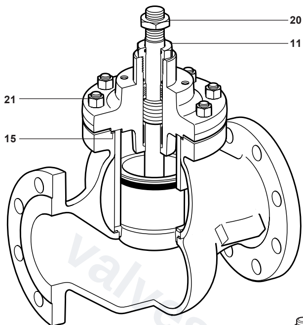
图24 平衡阀芯的阀门
