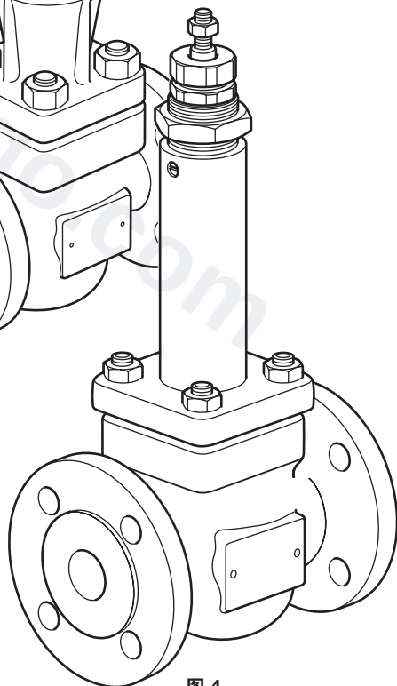
图 4 DN15 - DN100 KE, KEA, LE 和 LEA波纹管密封 (D)
