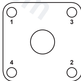
图5. 阀帽拧紧顺序
