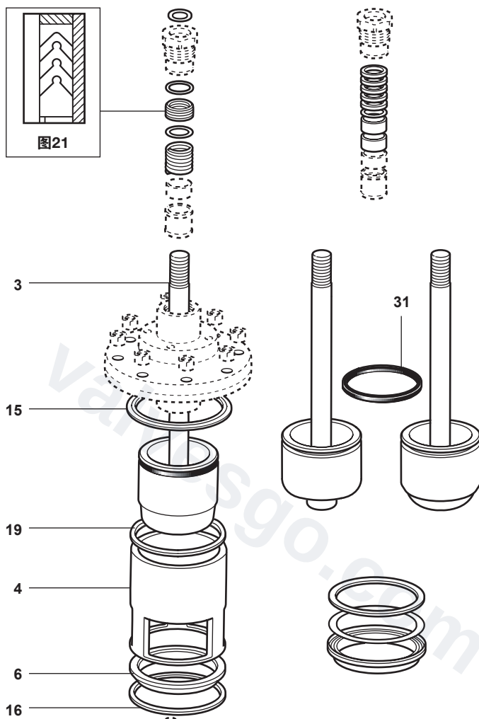
图22 平衡阀芯
