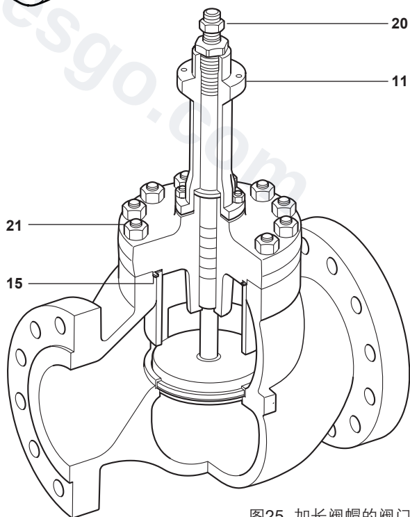
图25 加长阀帽的阀门
