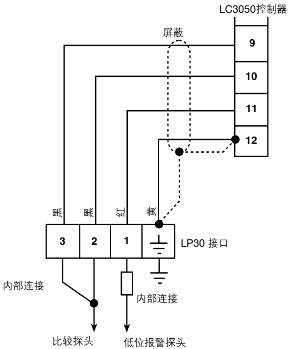
LP30低位报警接线详图
