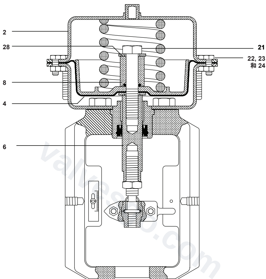
图10 PN9100E ( 弹簧伸张型 )
