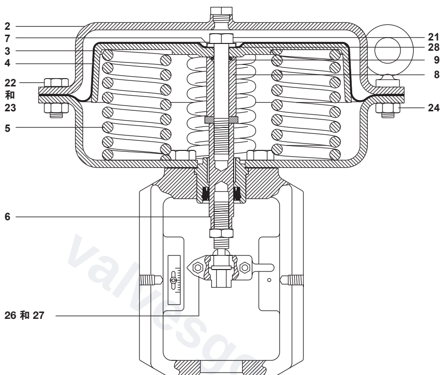
图11 PN9000R ( 弹簧回缩型 )
