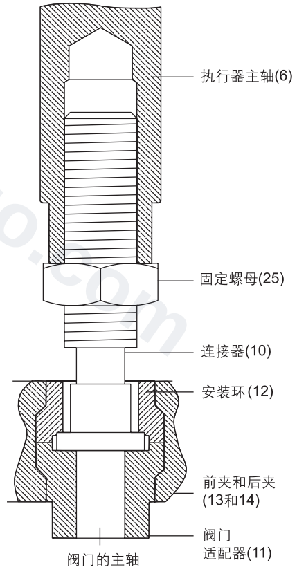
图6 执行器适配器，阀门适配器和连接器的安装
