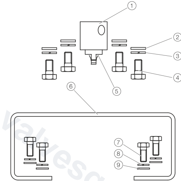
图12. 连接套件的组成部分
