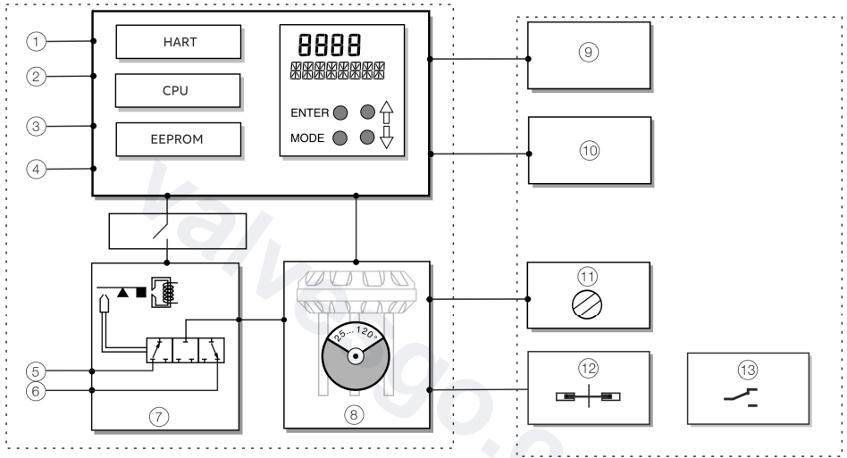
图1. 原理图
