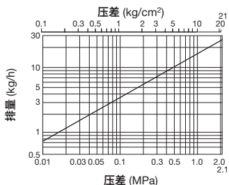
释放蒸汽 (阀门完全打开)
