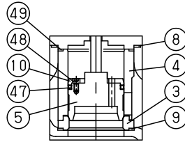
*D部断面図 (シール部)
