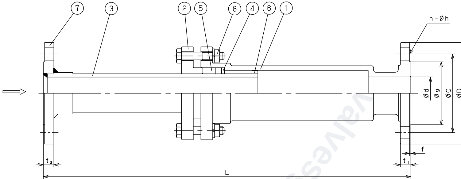
③スリーブ摺動部: 硬質クロームメッキ
