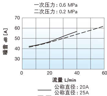
噪音特性图表
