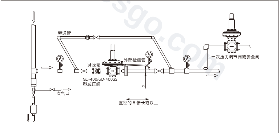
管道系统图例
