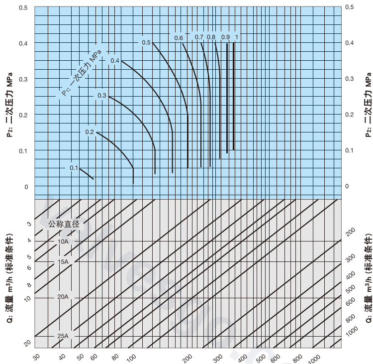
■ 公称直径选择图表（适用于空气）
