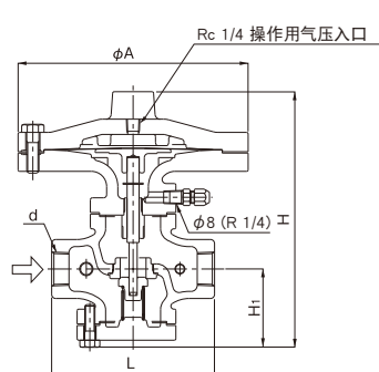
螺纹型
