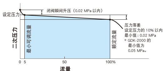
压力特性图表
