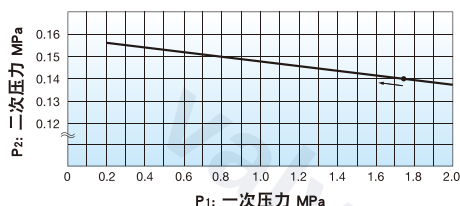
压力特性图表
