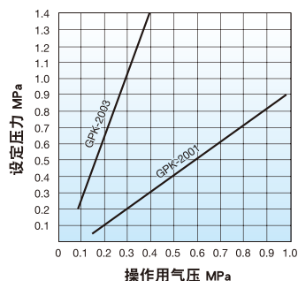
操作作用气压与设定压力图表
