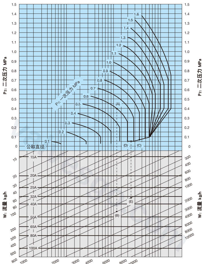
■ 公称直径选择图表 (适用于蒸汽)
