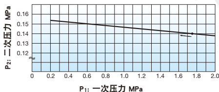
设定蒸汽减压阀出口侧的警戒用安全阀的压力
